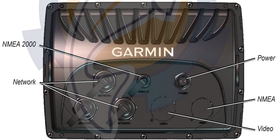
GPSMAP 5208 shown - Back
